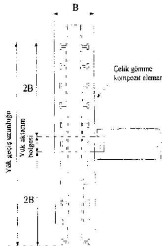
Şekil 12.9 – Yük aktarım bölgesi ve yük geçiş uzunluğu
