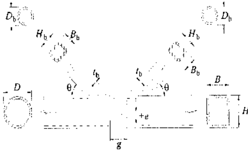
(a) Ara uzaklıklı K-birleşimi
