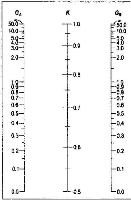
Şekil 6.1 – Yanal yerdeğiştirmesi önlenmiş sistemlerde burkulma boyu katsayısı, K
