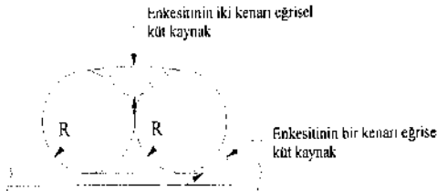
Şekil 13.2 – Enkesiti eğrisel kenarlı küt kaynaklar
