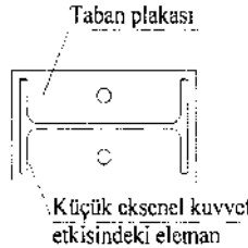
Şekil 13.10 – Küçük eksensel kuvvet etkisindeki elemanların ankrajı
