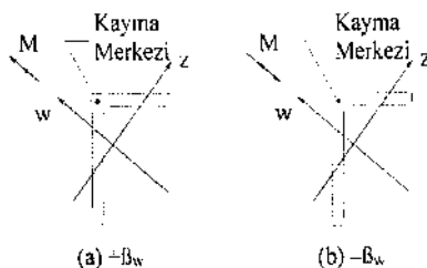
Şekil 9.2 - Eğilme momenti etkisindeki farklı kollu korniyerler için \beta_w işareti tanımları
