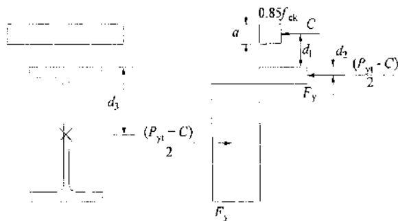
Şekil 12.2 - Kompozit kirişte pozitif eğilme momenti için genel plastik gerilme yayılımı
